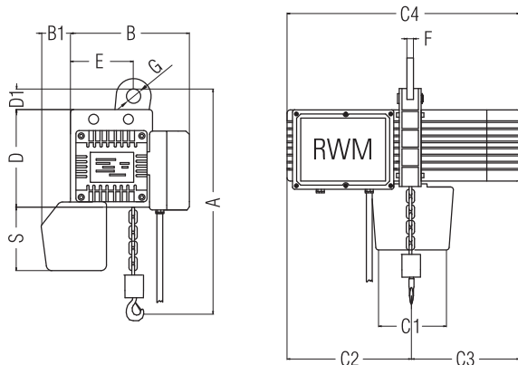
W Serija - Tip F (brez vozička)
