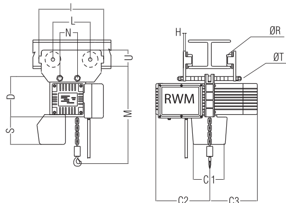
W Serija - Tip CS (potezni voziček)
